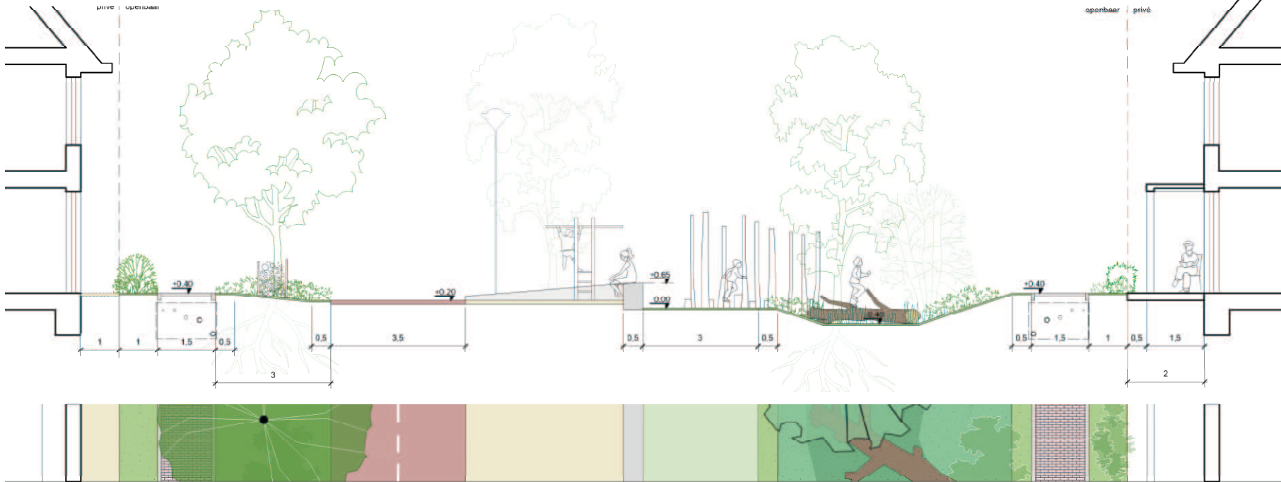
Doorsneden locatie
